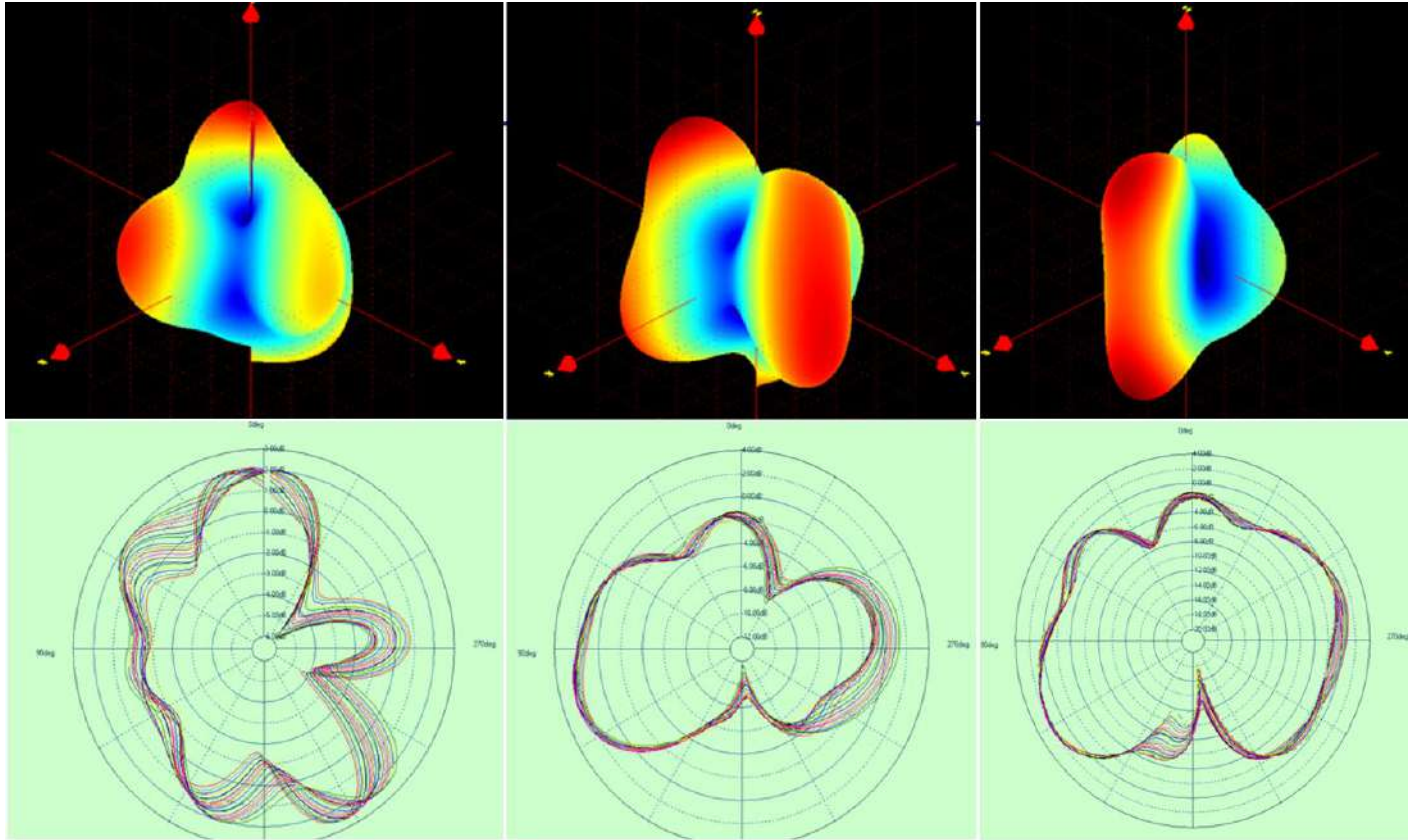
5GHz Pattern:
