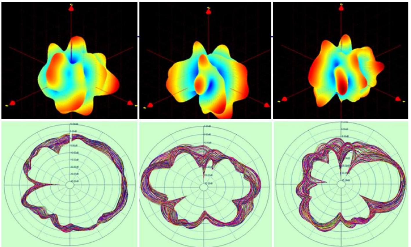
5GHz Pattern:
